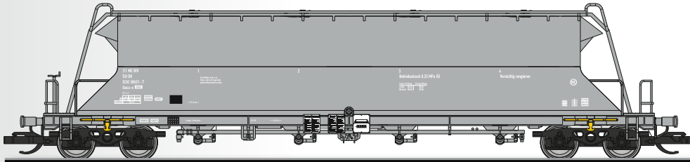
Selbstentladewagen Fcs 6450 der DR Hopper car Fcs 6450 of the DR
