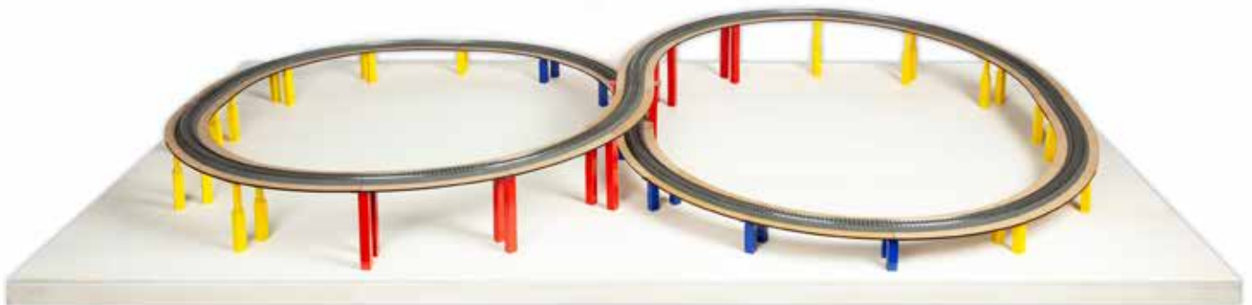
Die Pfeiler-Sets „unten“, „Steigung“ und „oben“ wurden in der Abbildung zum besseren Verständnis in den Farben blau, gelb und rot eingefärbt.
