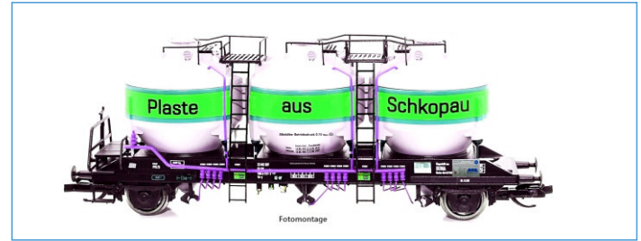
2-achsiger Silowagen Bauart Uc-y Museumswagen Chemiemuseum Merseburg (Epoche V) zum Transport von Kunststoffgranulate NW 52114 DC 2L TT 55,90 €
