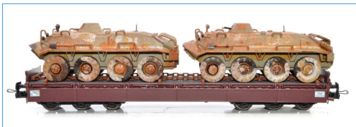
6-achsiger Schwerlastwagen Bauart Samms 4860 der DR (Epoche IV) Militärverkehr, beladen mit Schützenpanzern SPW 60 PB gealtert NW 22180 DC 2L H0 98,50 €
