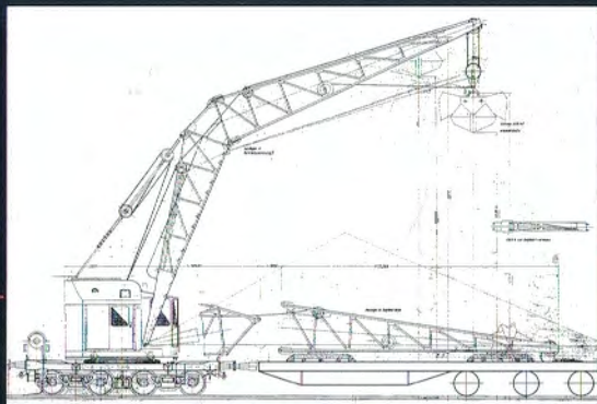
Bekohlungskran „EDK 6“
